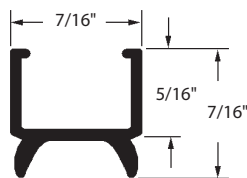
Moulure de contre-porte Storm Door Channel
