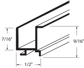
Rail pour contre-porte Storm Door Channel
