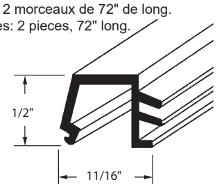
Moulure de contre-porte Storm Door Snap-In Glazing Stop
